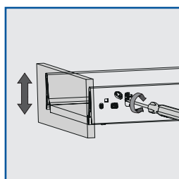
Regulación vertical: \pm 2.0 \text{ mm}
