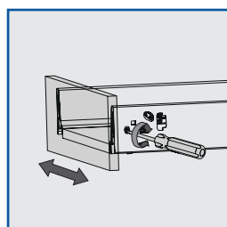
Regulación horizontal: \pm 1.5 \text{ mm}
